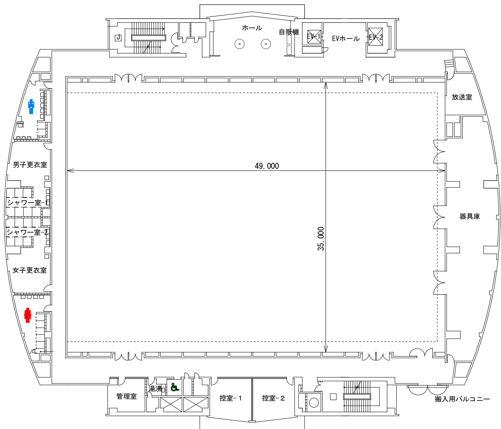
小アリーナ2F平面図 S=1/300 (atA3)
