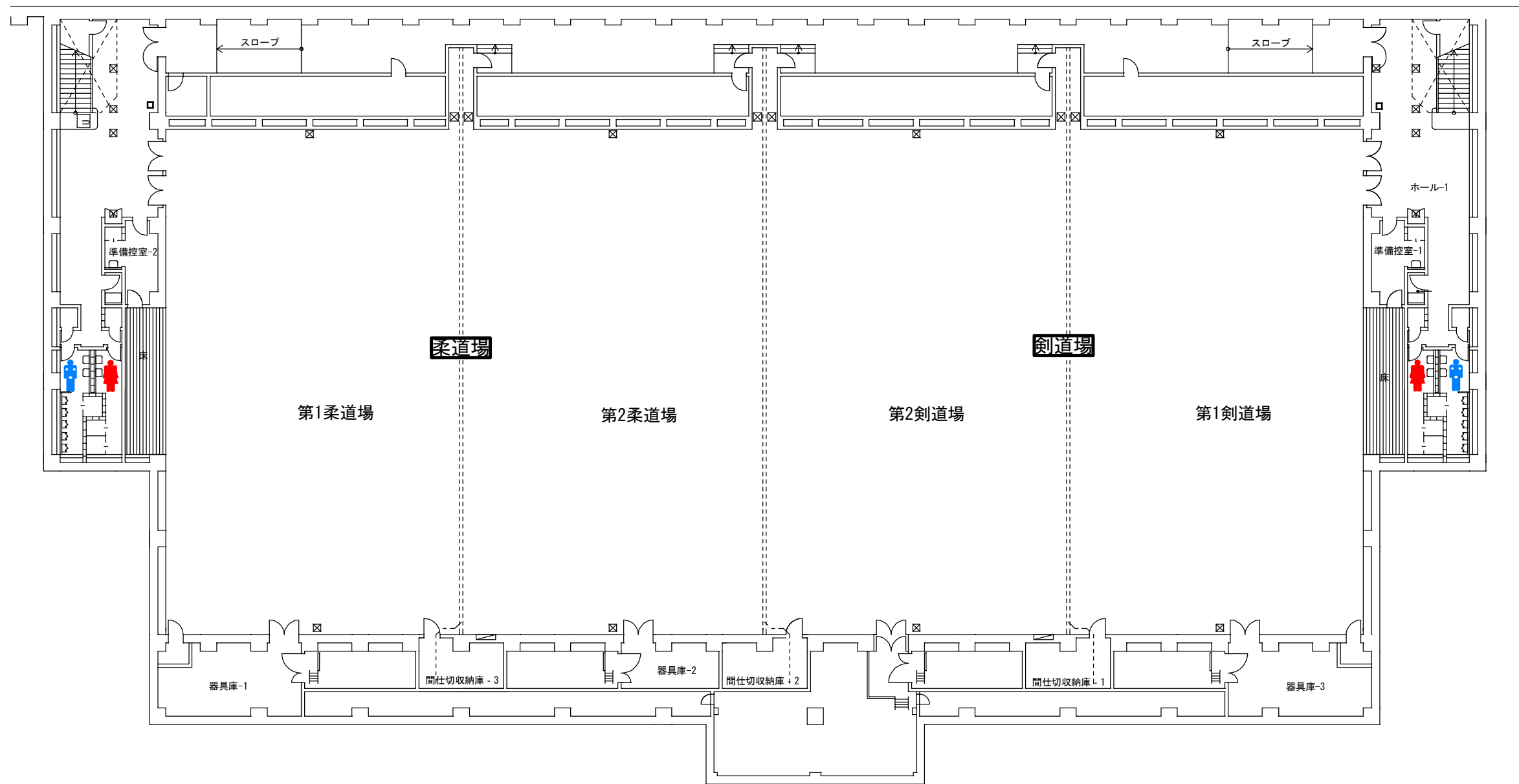
武道場B2F平面図 S=1/300 (atA3)
